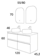
CARMEN 120 cm | 4 Tiroirs | Couleur 18 Poignée Incliné Aluminium Meuble + Plan K-Blanc + Vasques Circulaire K-Blanc
